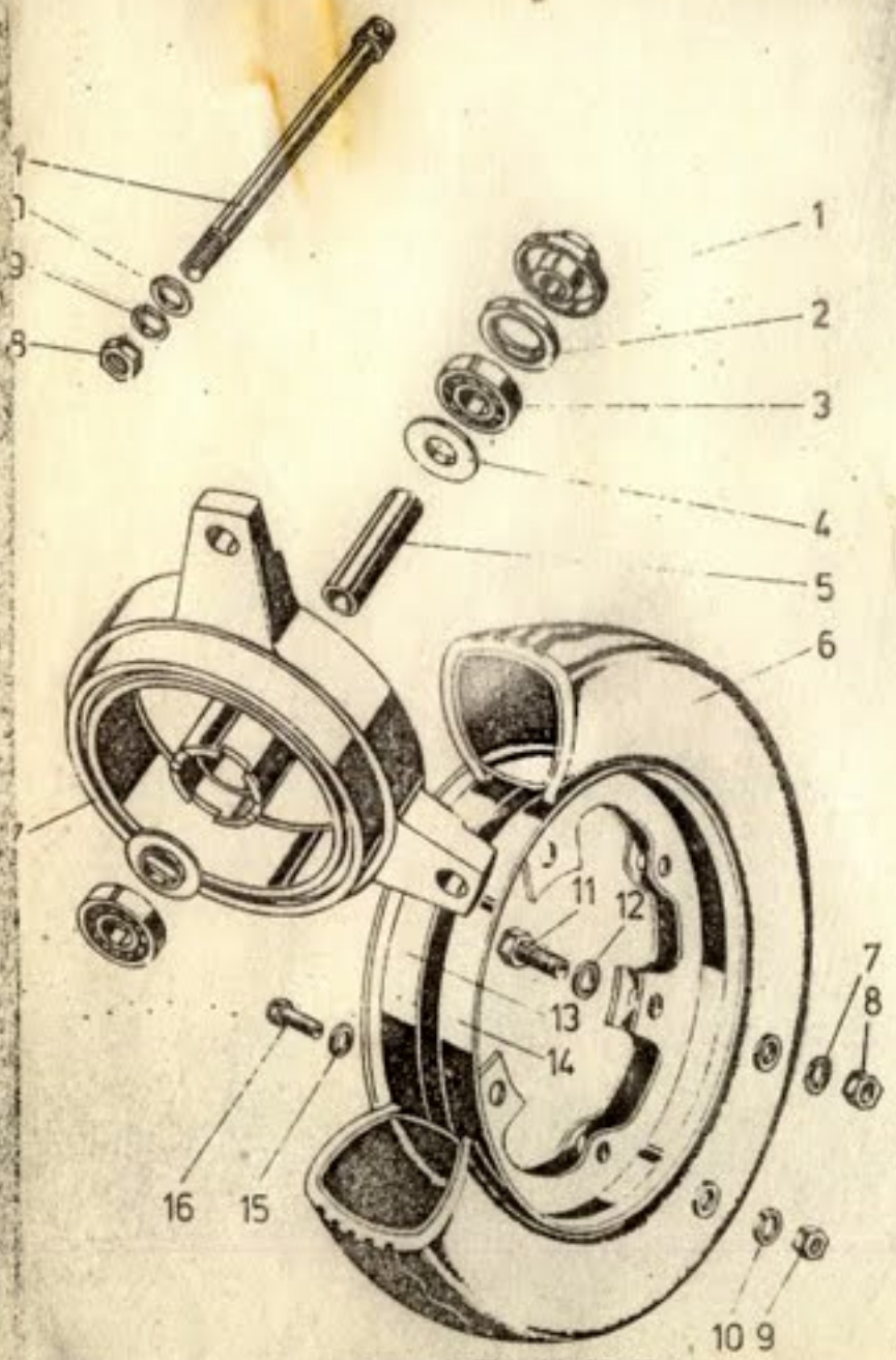
3. Колесо переднее в сборе 2.134-31.03.000
