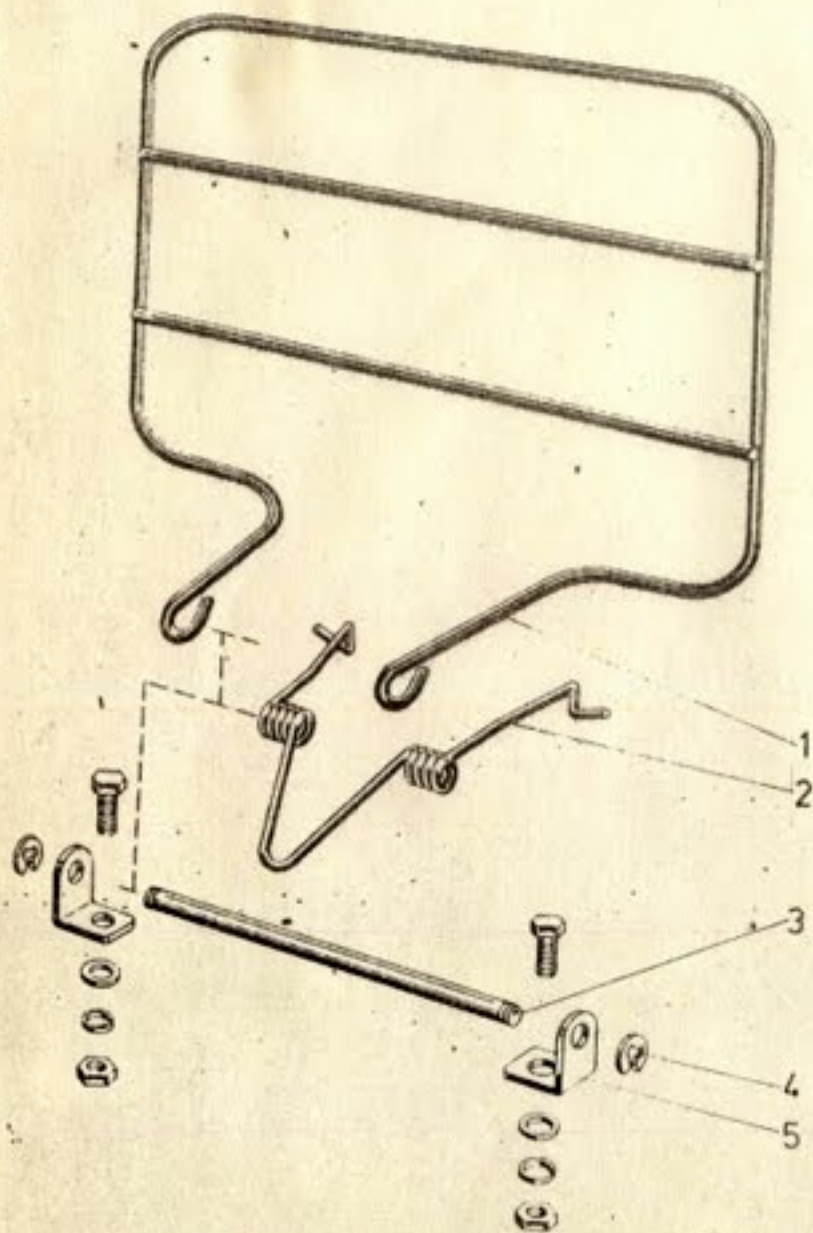
Рис. 26. Багажник передний 2-130-84.15.000 Б
