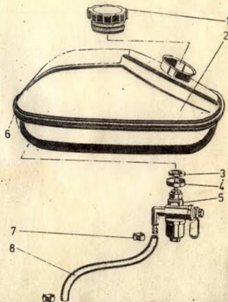
Рис. 1. Бак 2.134-11.01.000, кран с топливопроводом 2.134-11.04.000
