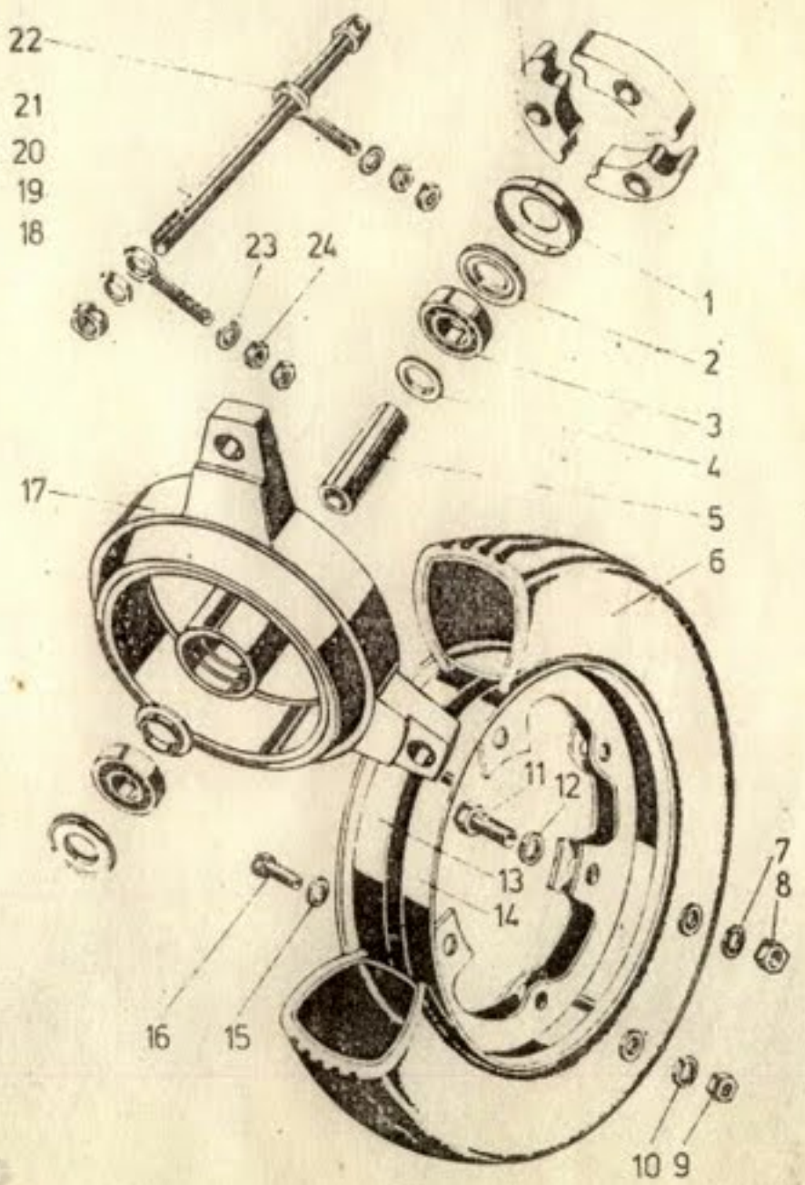
Рис. 9. Колесо заднее в сборе 2.134-31.04.000
