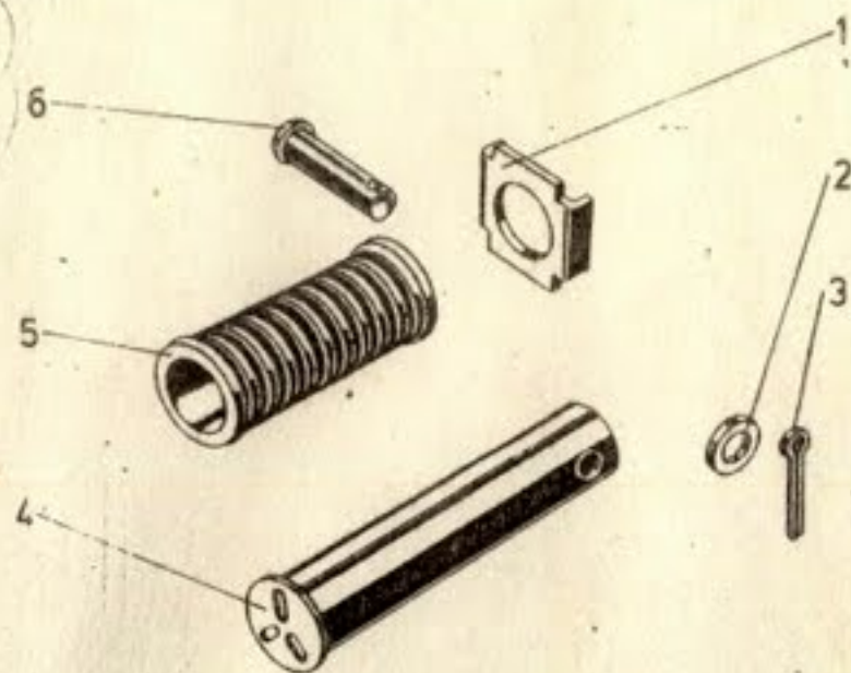
Рис. 27. Подножка 2.126-28.12.000
