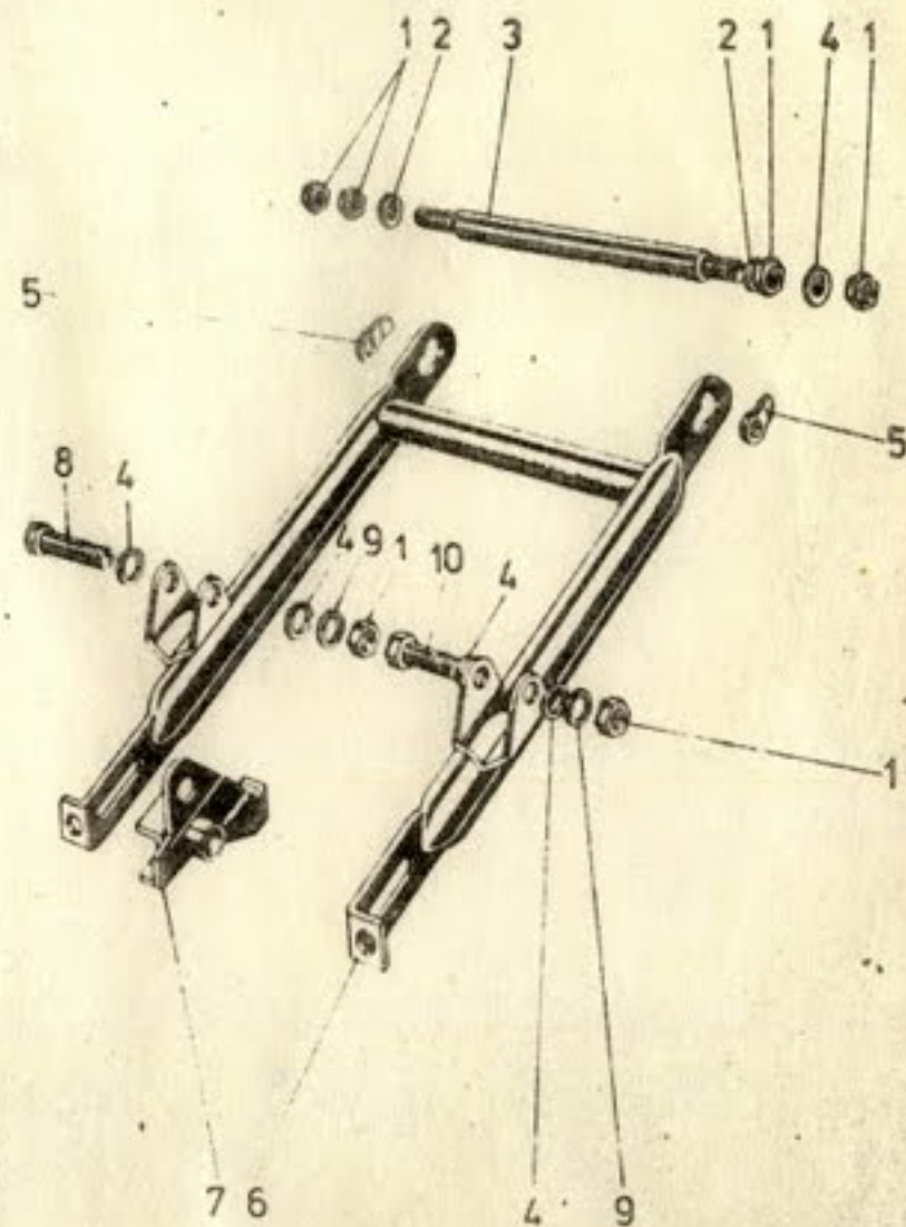
Рис. 5. Вилка задняя в сборе 2.134-28.05.000
